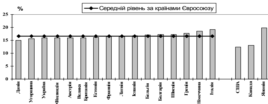
Рис. 2. Частка населення у віці 65 років і старше в Україні, країнах Європейського Союзу та деяких країнах інших регіонів світу у 2006 р. (Джерело: Europe in figures-2006. — Eurostat yearbook, 2006)
