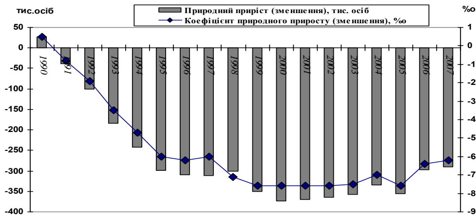
Рис. 1. Природний приріст (зменшення) та коефіцієнт природного приросту (зменшення) населення в Україні у 1990 – 2007 рр. (Джерело: дані Державного комітету статистики України)
