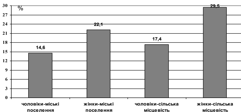
Рис. 3. Частка населення у віці 60 років і старше за типом поселення та статтю в Україні (на початок 2008 р.; джерело: розрахунки за даними Державного комітету статистики України)
