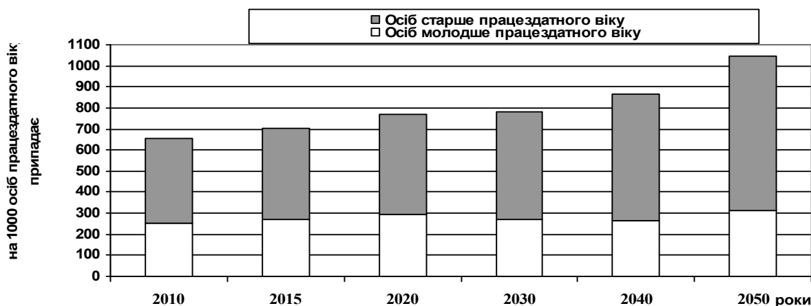
Рис. 4. Демографічне навантаження на населення працездатного віку в Україні на період до 2050 р. (джерело: розрахунки за середнім варіантом демографічного прогнозу України на період до 2050 р., розробленого Інститутом демографії та соціальних досліджень НАНУ)
