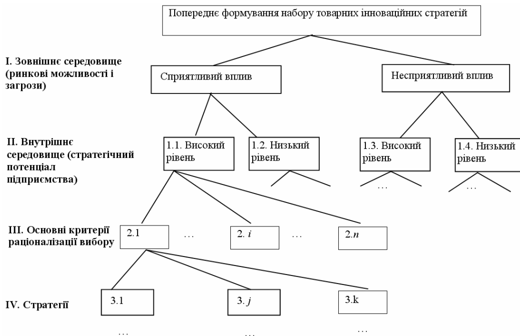
Рис. 1. Ієрархічна структура вибору стратегій
