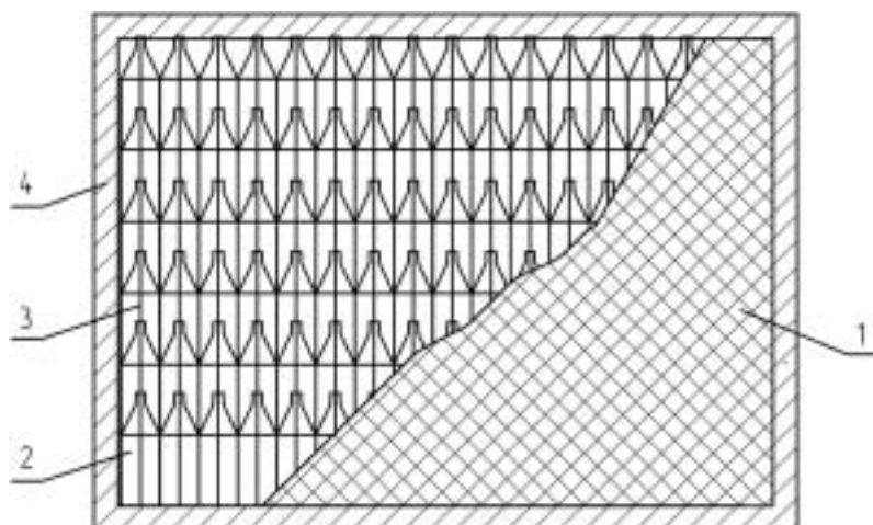
Рис. 1. Теплоізоляційна панель: 1 – каркас; 2 – пластикові пляшки з відрізнаним дном; 3 – дріт; 4 – захисний повітронепроникливий корпус
