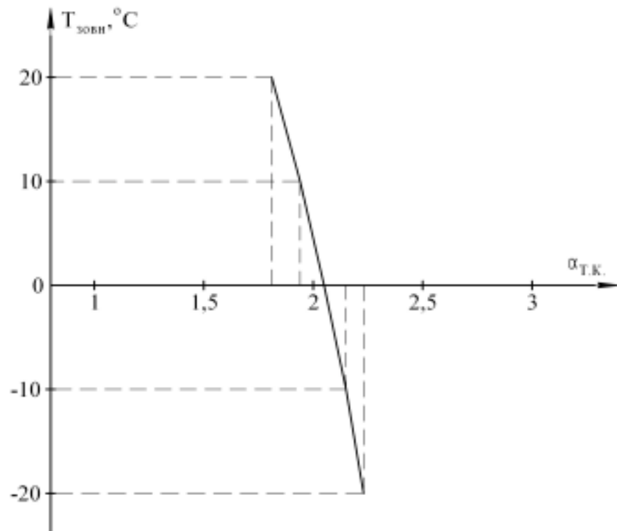
Рис. 4 Графічне зображення залежності коефіцієнта теплопереходу конвекцією від температур зовнішнього середовища Для герметичних повітряних прошарків теплоізоляційних конструкцій (рис. 1, 2) за результатами
