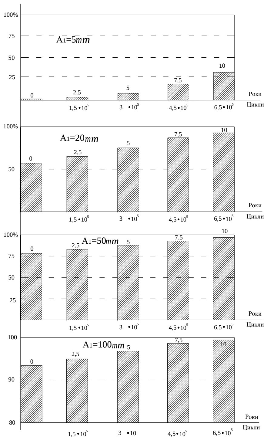
Рис. 5. Порівняльна характеристика впливу початкової вимушуючої амплітуди коливань на відносне проковзування системи цемент-сталь. Початкове нормальне навантаження на зразки P_n=100\text{ Н} (0,2 МПа).
