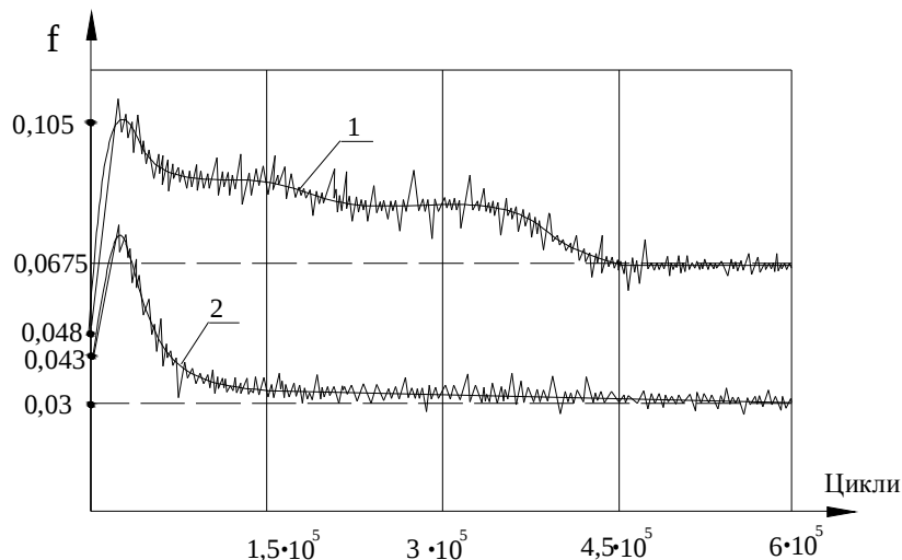
Рис. 10. Залежність коефіцієнта тертя в парі поліетилен – сталь від числа циклів навантаження. 1 – на сухо, 2 – в середовищі замінильника синовіальної рідини.
