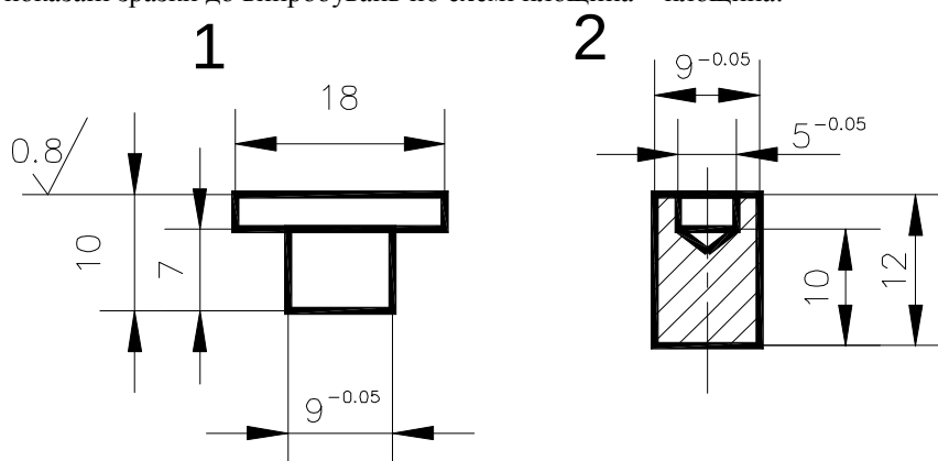
Рис. 4. Зразки до випробування на відносну рухомість та фреттингостійкість. 1 – цемент, 2 – сталь
