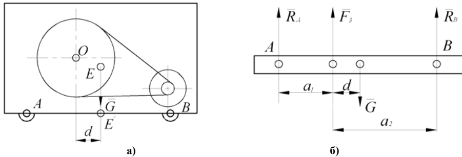
Рис. 3. Визначення положення центра ваги
