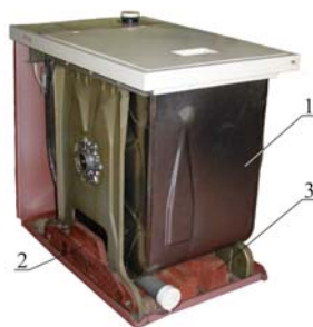
Рис. 1. Пральна машина "Айша" 1 – пральна машина "Айша"; 2 – вантаж масою 6 кг; 3 – вантаж масою 14 кг
