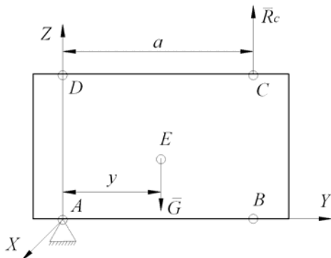
Рис. 2. Визначення положення центра ваги
