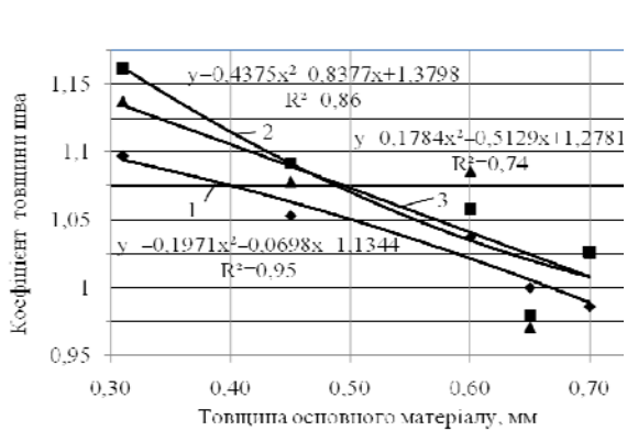
Рис. 5. Залежність коефіцієнта товщини шва від товщини основного матеріалу: 1) шов 1; 2) шов 2; 3) шов 3
