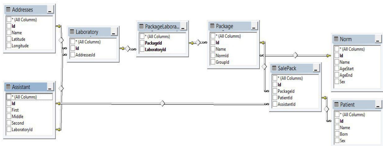
Рис. 2. Структурна схема бази даних консолідованого ресурсу
