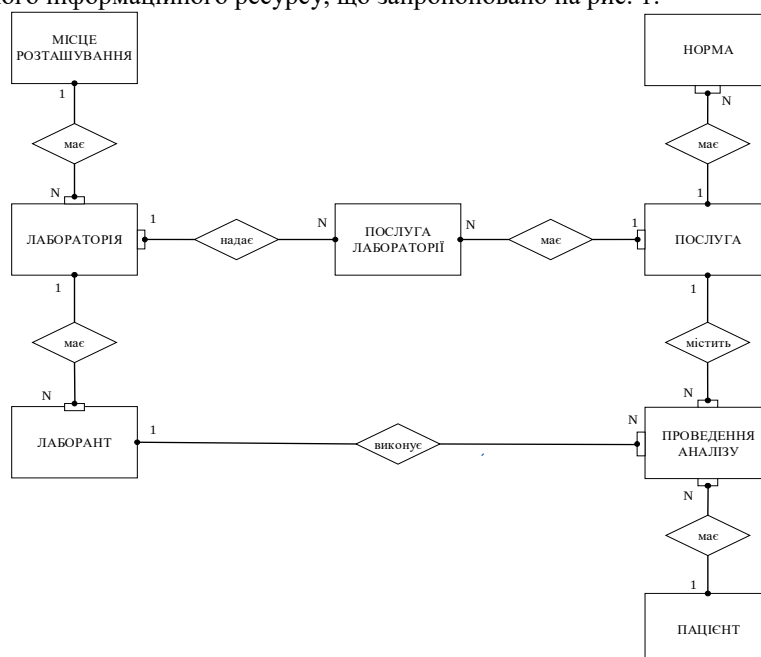
Рис. 1. ER-модель консолідованого інформаційного ресурсу для аналізу ринку надання послуг медичними лабораторіями України
