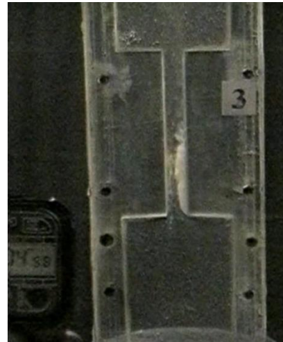
Рис. 12. Фотографія прозорого каналу з рідиною, що коливається в момент втягування рідини у камеру пульсації: виникнення кавітаційної каверни та кавітаційних пухирців при збільшенні частоти коливань до 10 Гц
