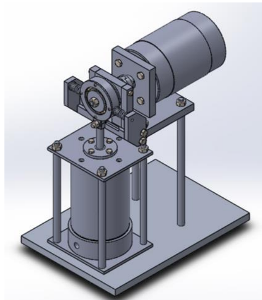
Рис. 2. Просторова 3D-модель вібраційної машини
