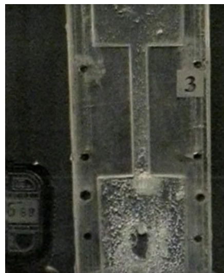
Рис. 10. Фотографія прозорого каналу з рідиною, що коливається в момент втягування рідини у камеру пульсації: виникнення кавітаційної каверни та кавітаційних пухирців при збільшенні частоти коливань до 16 Гц; поява великої кавітаційної каверни
