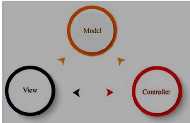
Рис. 1. Зміст веб-фреймворка.
