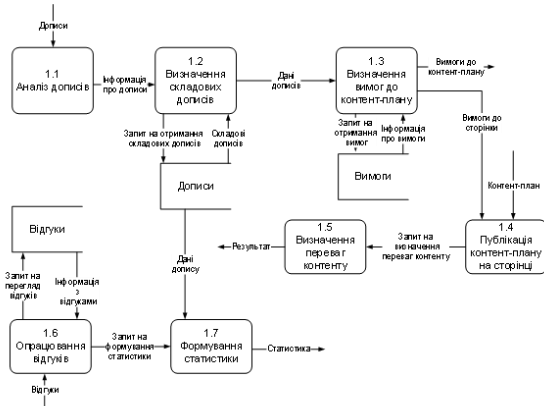
Рис. 2. Деталізація першого рівня DFD-моделі
