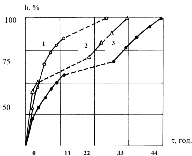
Рис. 1. Кінетика дифузії танідів у дерму обертаючого барабана, – – – стан покою)
