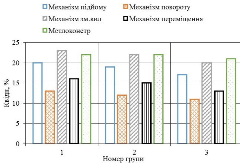
Рис. 3. Розподіл коефіцієнтів відмов Квідн (а) та часу відновлення Квідн (б) вузлів порталних кранів «Ганц»
