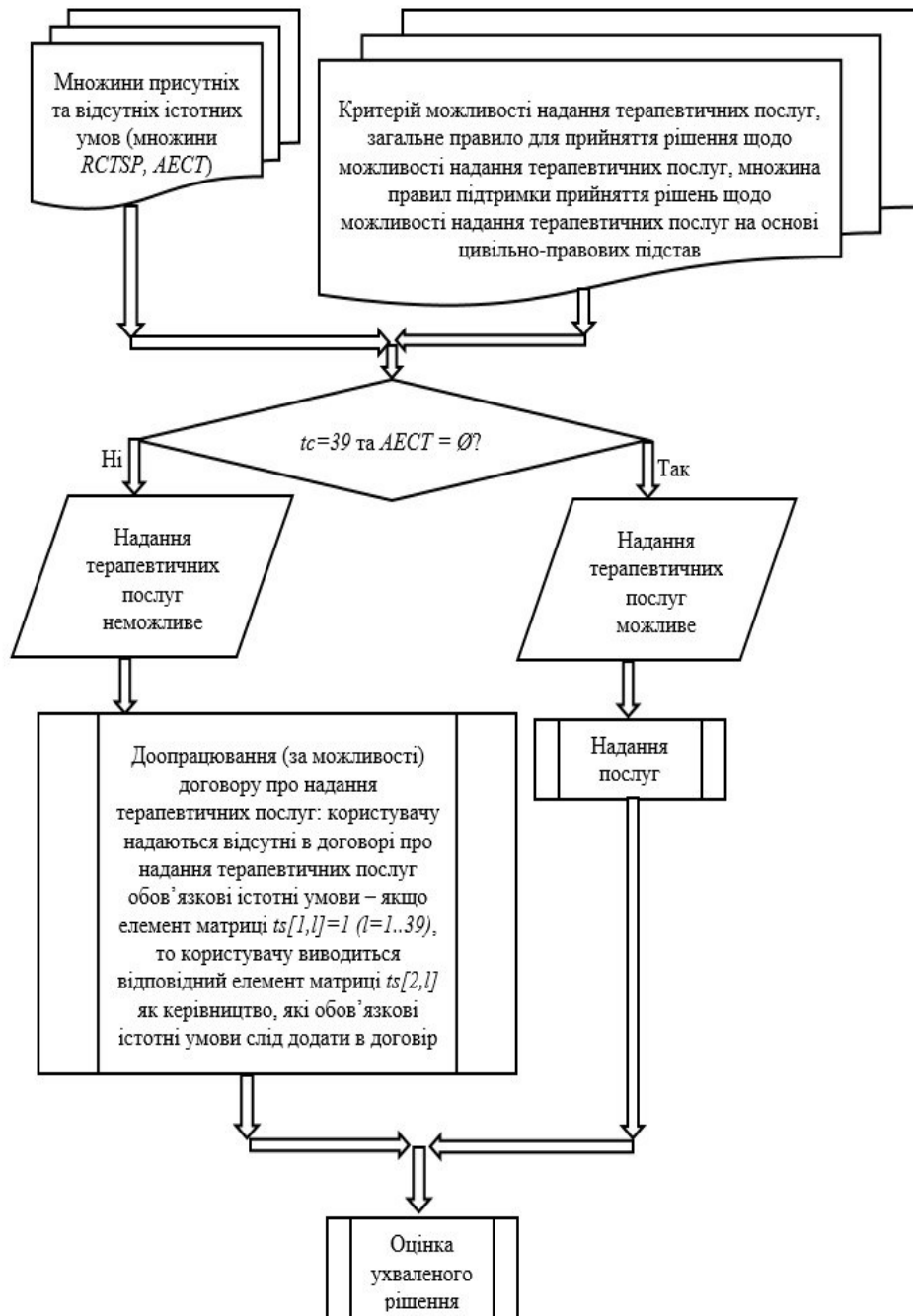
Рис. 3. Схема методу підтримки прийняття рішень щодо можливості надання терапевтичних послуг на основі цивільно-правових підстав
