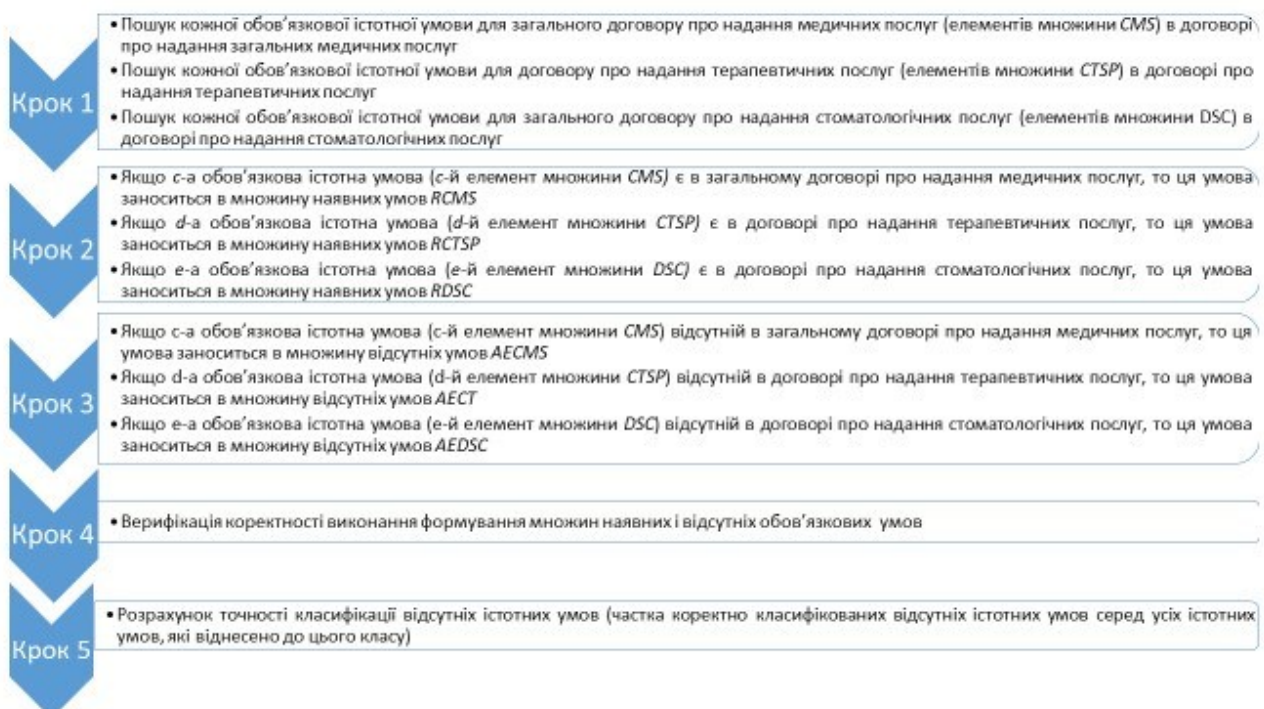
Рис. 1. Схема методу семантичного аналізу (парсингу) природомовних загального договору про надання медичних послуг та похідних від нього договорів – договору про надання терапевтичних послуг і договору про надання стоматологічних послуг
