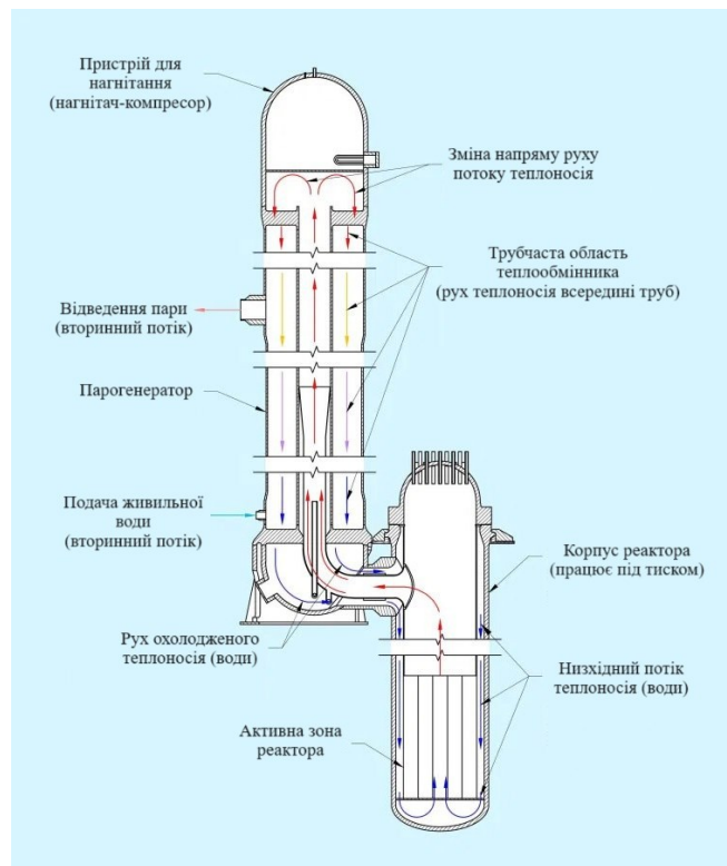
Рис. 2. Загальний вигляд та складові реактора SMR-160
