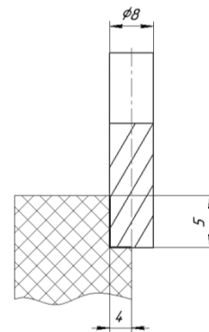
Рис. 2. Схема оброблення - уступ
