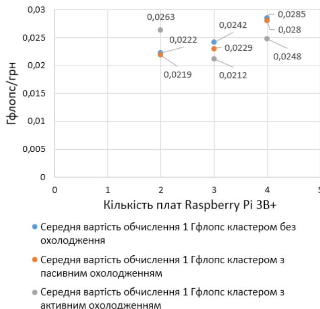
Рис. 4. Середні значення вартості обчислення 1 Гфлопс кластерною системою на базі одноплатних комп’ютерів Raspberry Pi 3B+ при різній кількості плат Raspberry Pi 3B+ в ній та при різних підходах до охолодження кластера
